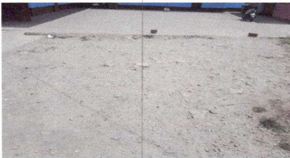
Foto 4: Reparación de planchas de concreto, de patio
